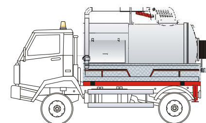
COMBI 1000/500/60 ΣΥΝΘΕΤΟ ΑΠΟΦΡΑΚΤΙΚΟ ΣΥΓΚΡΟΤΗΜΑ
