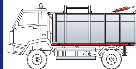
SMV 17 ΑΝΑΡΡΟΦΗΤΗΣ ΦΥΛΛΩΝ ΜΙΚΡΟΑΠΟΡΡΙΜΜΑΤΩΝ
