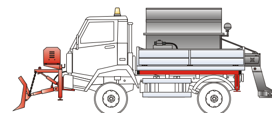
SWC 40 MP ΠΡΕΣΣΑ ΑΠΟΡΡΙΜΜΑΤΩΝ ΧΩΡΗΤΙΚΟΤΗΤΑΣ 4m³
