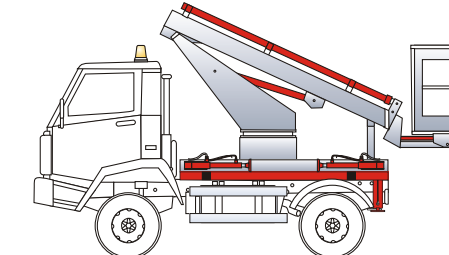
TLC 13,5, 15 ΤΗΛΕΣΚΟΠΙΚΟ ΚΑΛΑΘΟΦΟΡΟ ΟΧΗΜΑ ΜΕ ΥΨΟΣ ΕΡΓΑΣΙΑΣ 13,5 ή 15m
